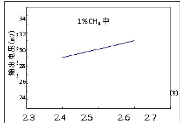
图 10：灵敏度电压波动特性曲线
