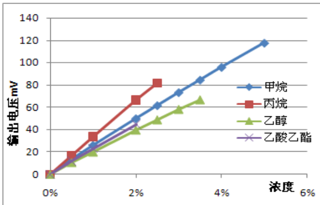
图3：灵敏度曲线
