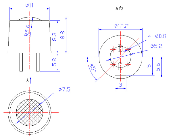
图1：传感器外形结构
